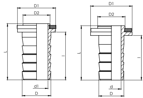
Mit Dichtungsfixierung
